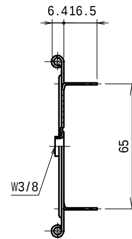
A-A断面図 (OF-S35S2 L)
